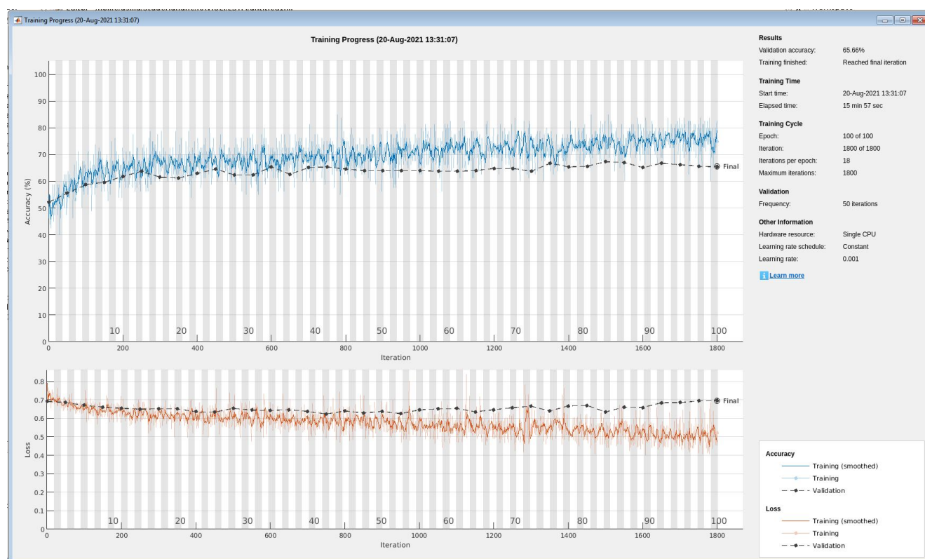
Fig 4.10 – Représentation de la fonction de perte et de la précision des ensembles de validation et de test de la deuxième base.
